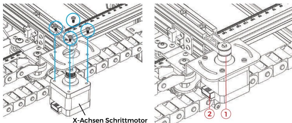
X-Achsen Schrittmotor
