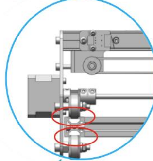
Eccentric nut
